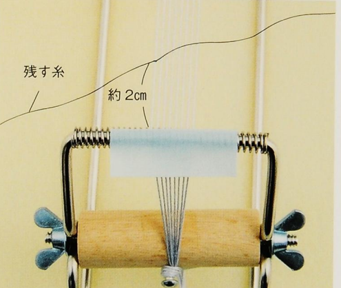
1 よこ糸(260cm)を15cm残し、左端のたて糸のバネから約2cm離れたところに結びます。
