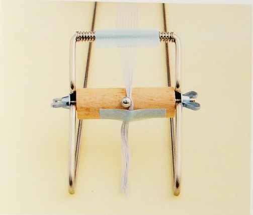
7 8本のたて糸をひとまとめにし、止め棒に2回巻きつけて巻棒にマスキングテープでとめます。
